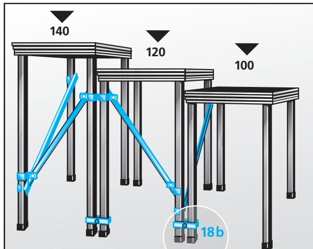
20 Bühnenaufbau mit Verbindungsstreben und -klammern Assemblage de podium avec traverse et brides Assembling of platforms with cross rail and clamps
