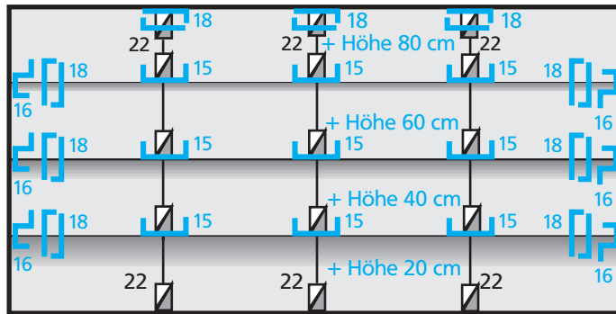
14 Aufstellungsbeispiel Höhe 20 - 80 cm Exemple de configuration hauteur 20 - 80 cm Configuration example height to 20 - 80 cm
